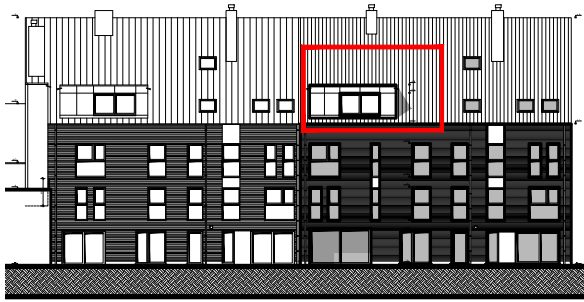
ACHTERGEVEL
